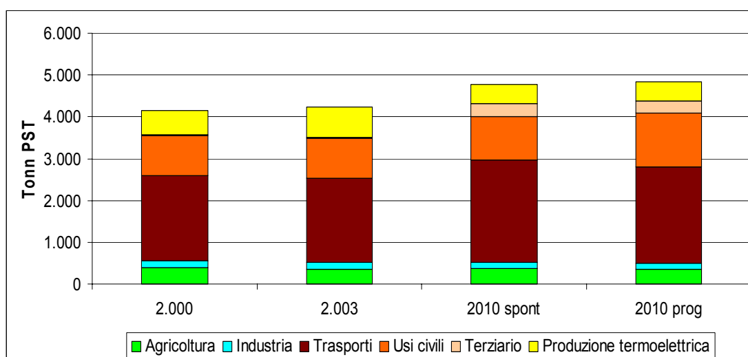
Figura 6: Scenari di emissione di PST al 2010 (t).
