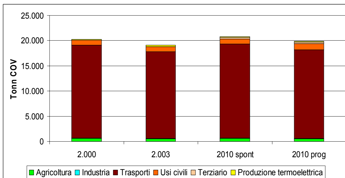
Figura 5: Scenari di emissione di COV al 2010 (t).
