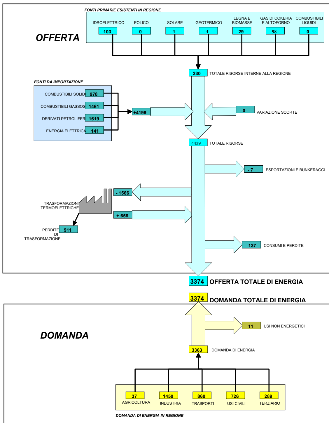
Figura 1: Schema semplificato del sistema energetico regionale al 2003
