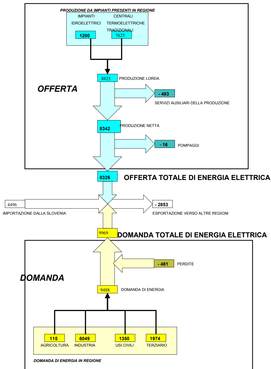
Figura 2: Bilancio elettrico regionale per l'anno 2003.
