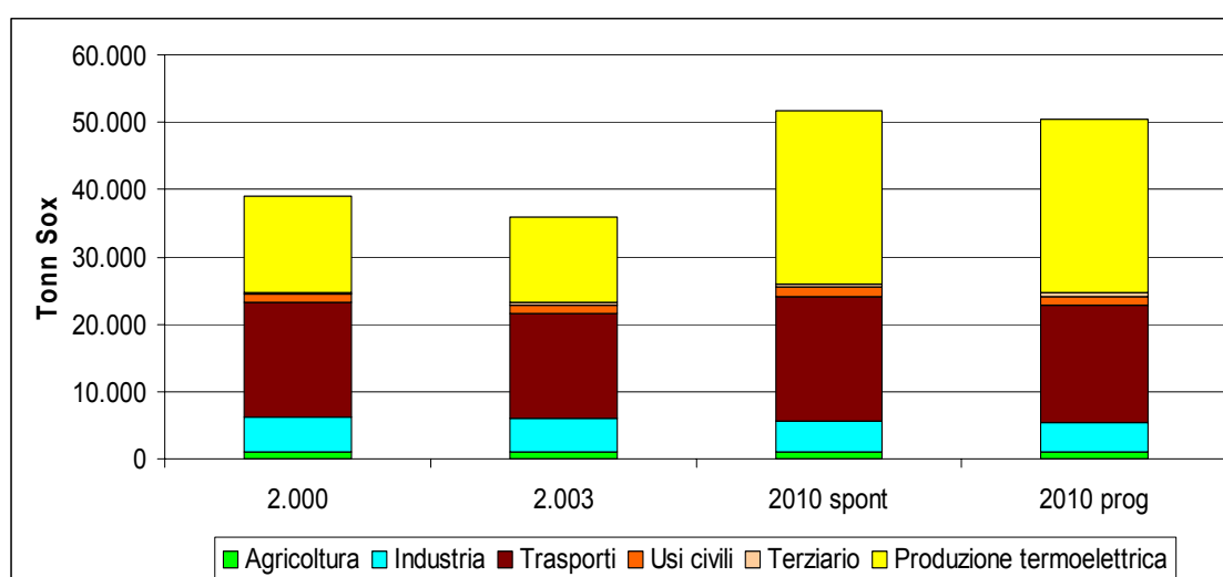
Figura 3: Scenari di emissione di NOx al 2010 (t).
